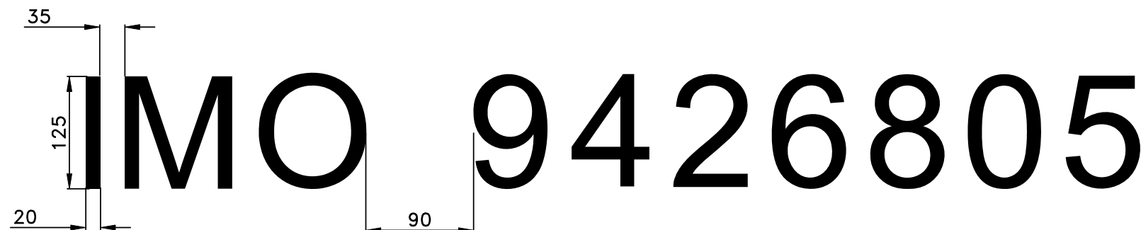
机舱标志字样尺寸 (H2432)
